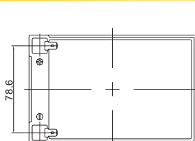
F2 Terminal
